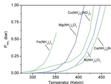
Figur 5. Sammenligning af ammoniaktrykkene over forskellige metalaminer. Alle de viste materialer har ligevægtstryk, der både giver en acceptabel sikkerhed og mulighed for at desorbere ammoniakken ved passende lave temperaturer. Molmasserne af de fem salte er meget forskellige, og magnesiumsaltet er den bedste kandidat, fordi det har den laveste molmasse og dermed den største vægtprocent brint.
